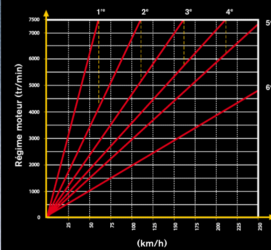
Boîte de vitesses manuelle à 6 rapports courts
