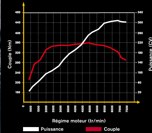
2007 : nouveau moteur V6 3,5
